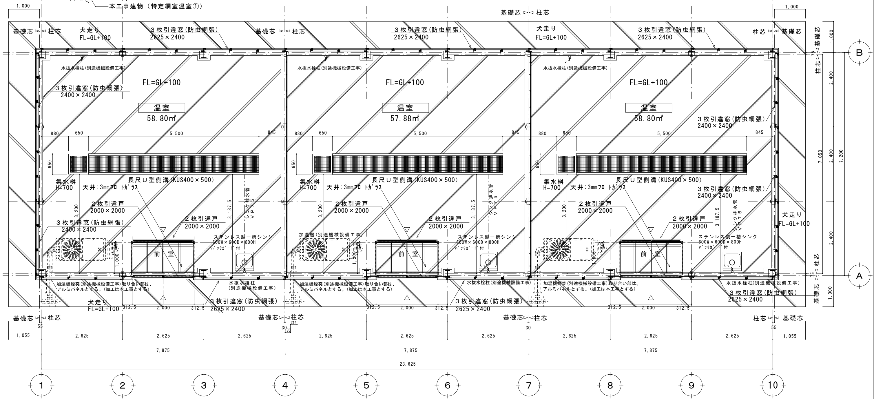
平面図 1/50
